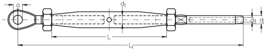
NIRO Wantenspanner mit Auge und Terminal Standard
