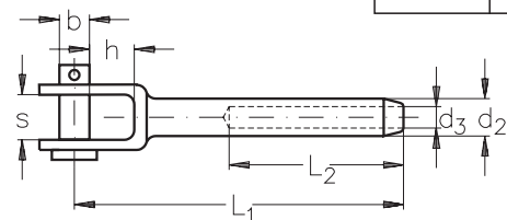
ASS Mini-Gabelterminal
