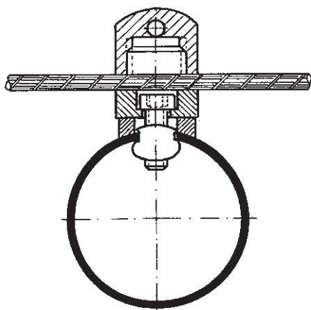
Befestigung der ASS Anschraubklemme an einem Rundrohr mit ASS Radienscheibe. Fixing of the ASS Attaching clip to a round post with ASS Special Washer.
