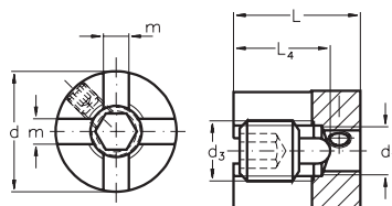
NIRO Kreuzklemme, einfach mit Wandanschluß M 8
