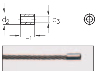
montiert assembled
