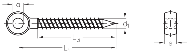
NIRO Augenschraube DIN 444 mit Holzgewinde, rechts
