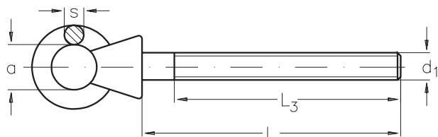
NIRO Ösenschaube lange Ausführung, Rechtsgewinde
