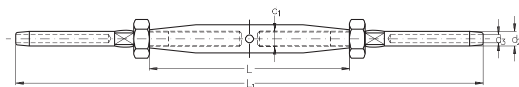
NIRO Wantenspanner mit zwei Terminals Standard
