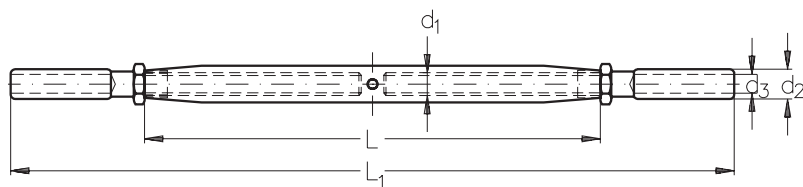
ASS Super-Mini-Wantenspanner mit zwei Terminals, lange Ausführung
