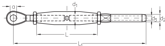
ASS Mini-Wantenspanner mit Auge und Terminal
